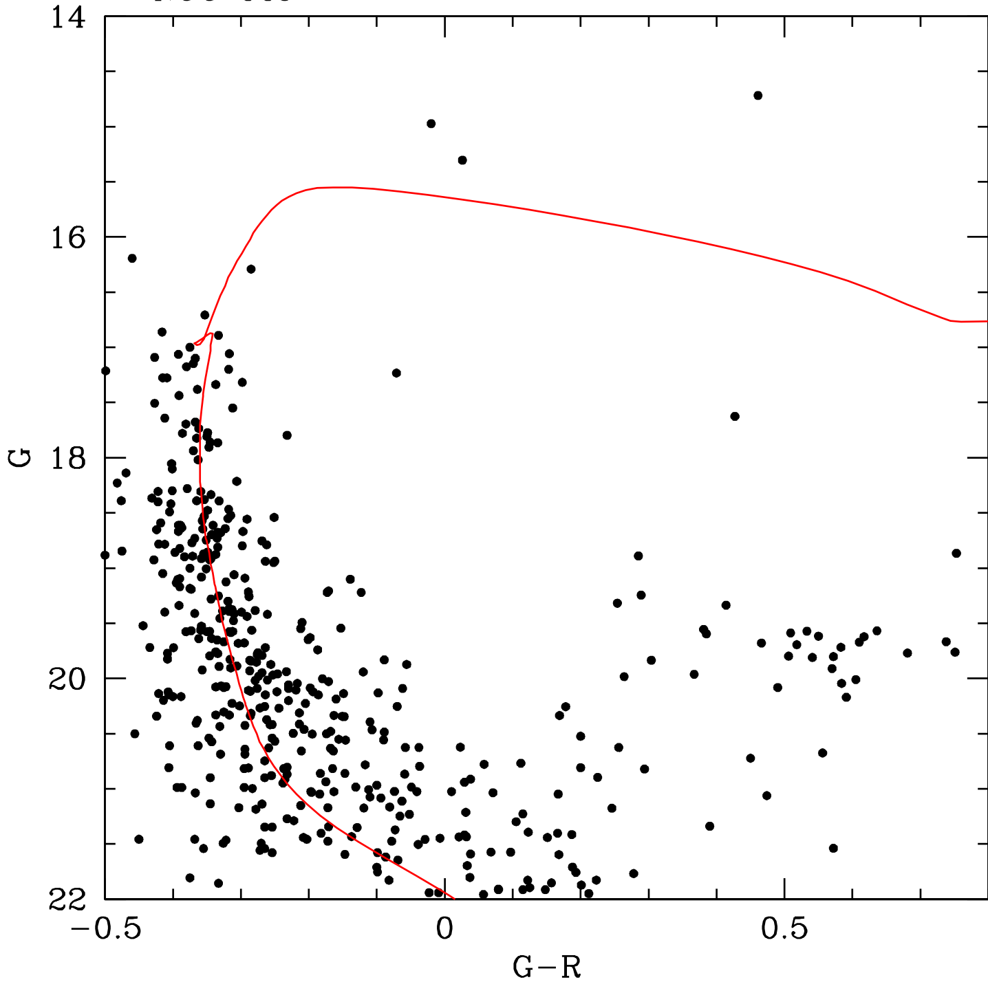
NGC 220
