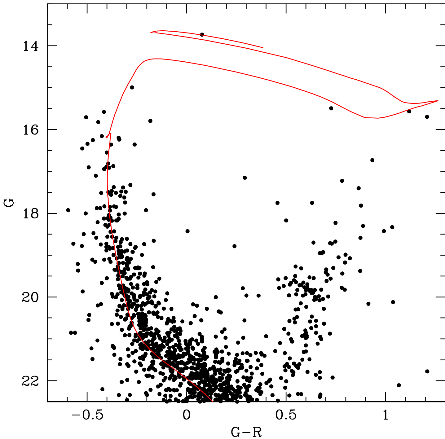
NGC 306
