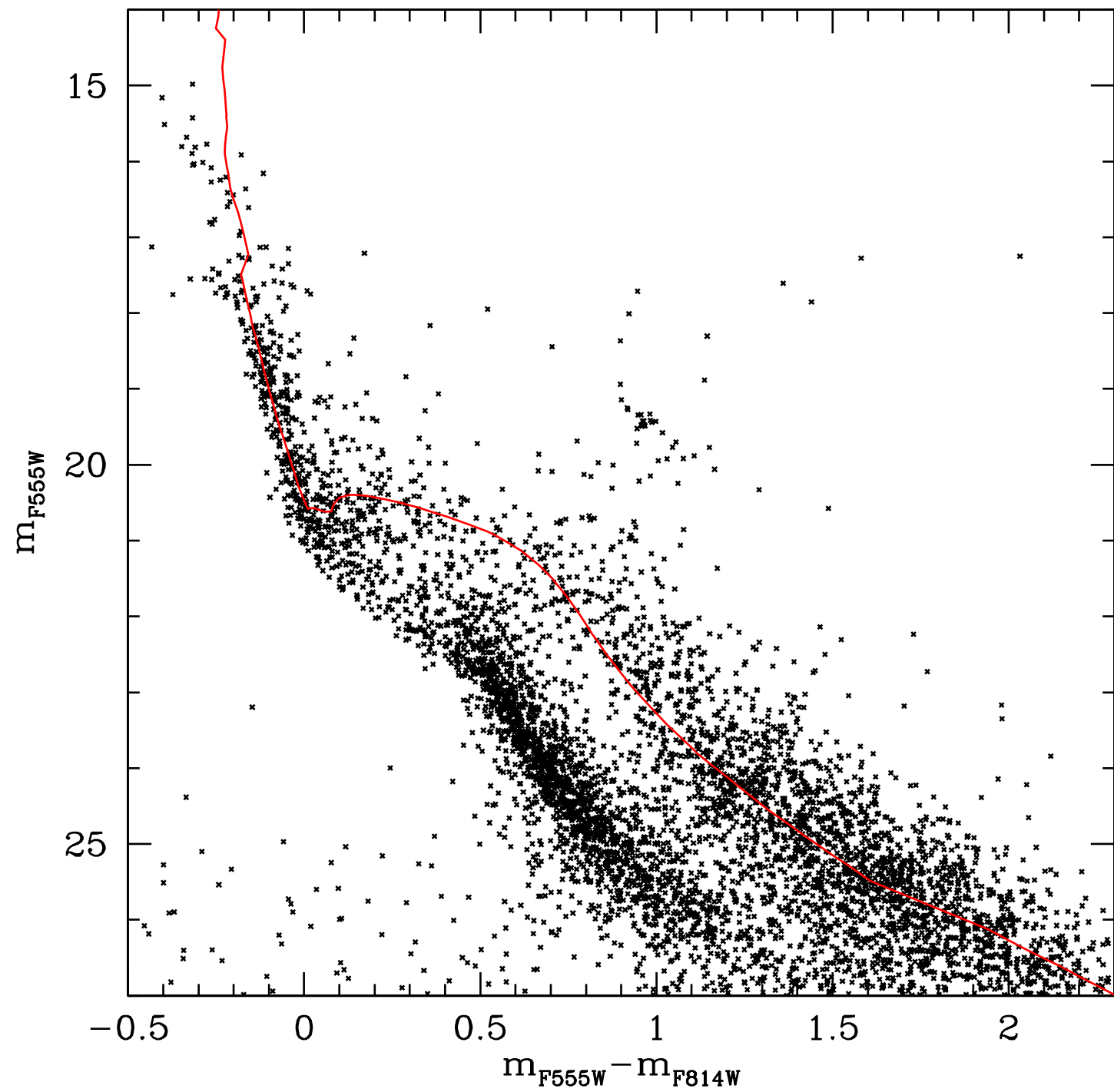
NGC 346
