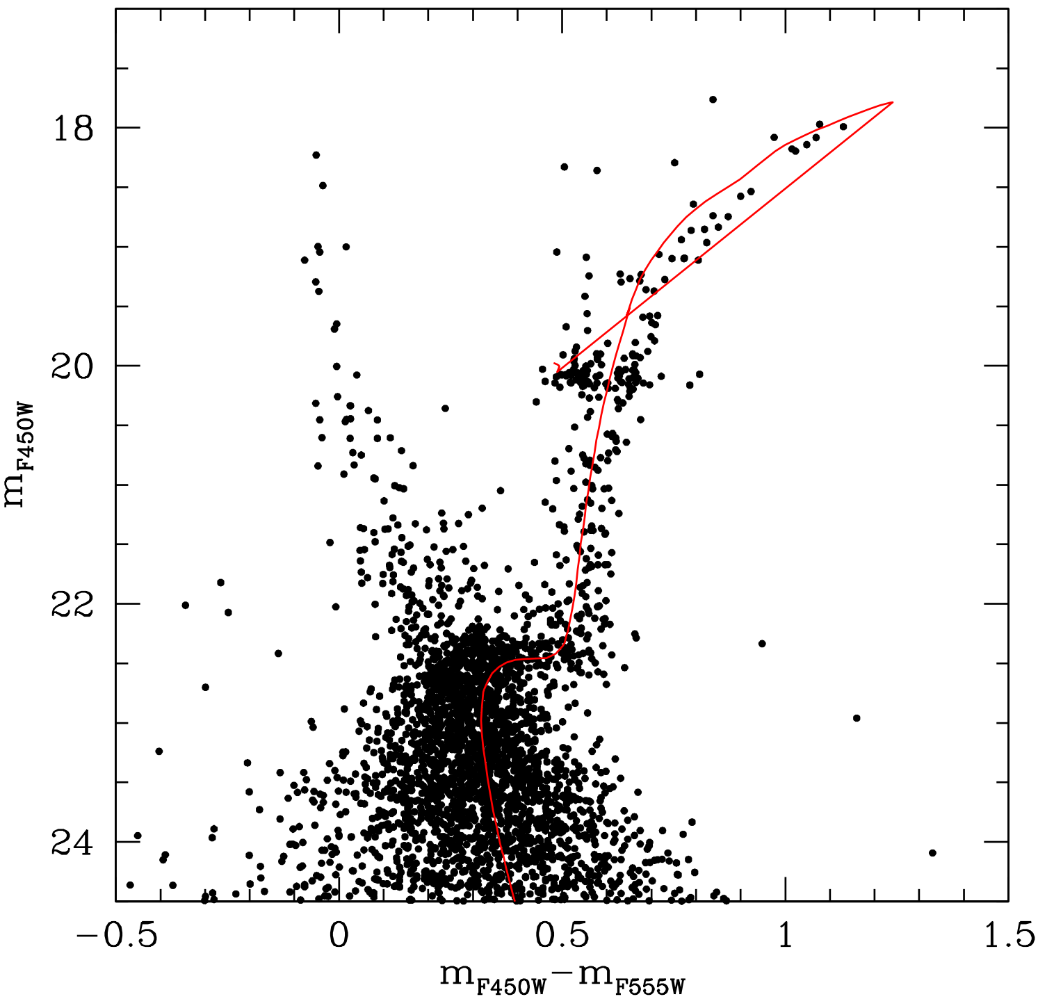
NGC 361
