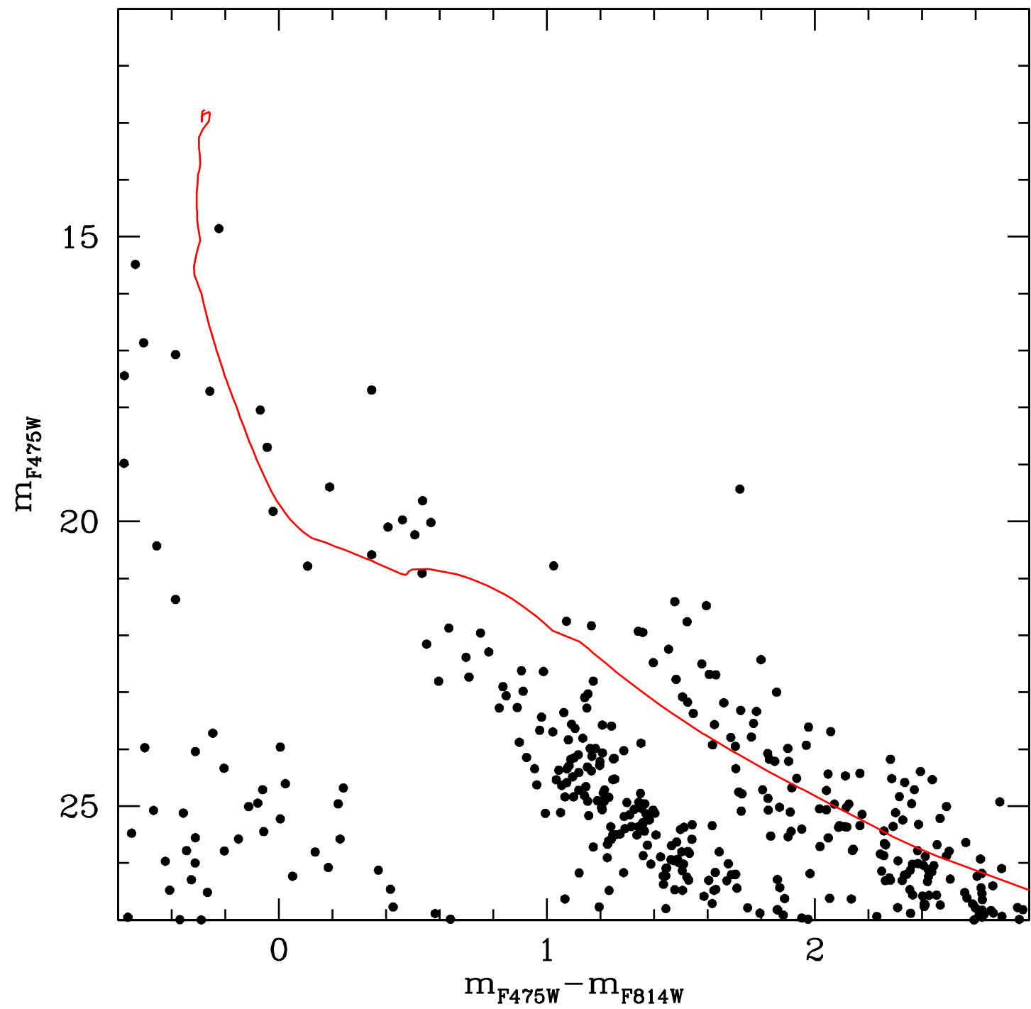
NGC 460
