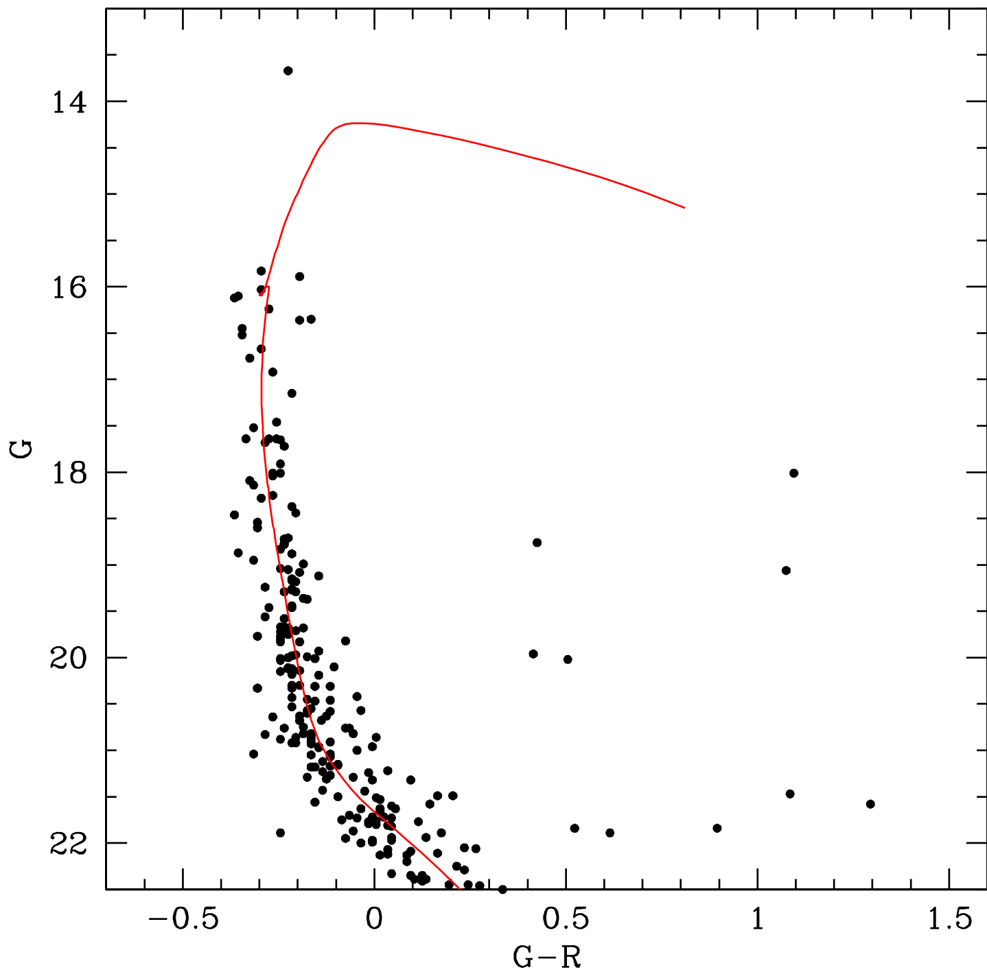
NGC 796
