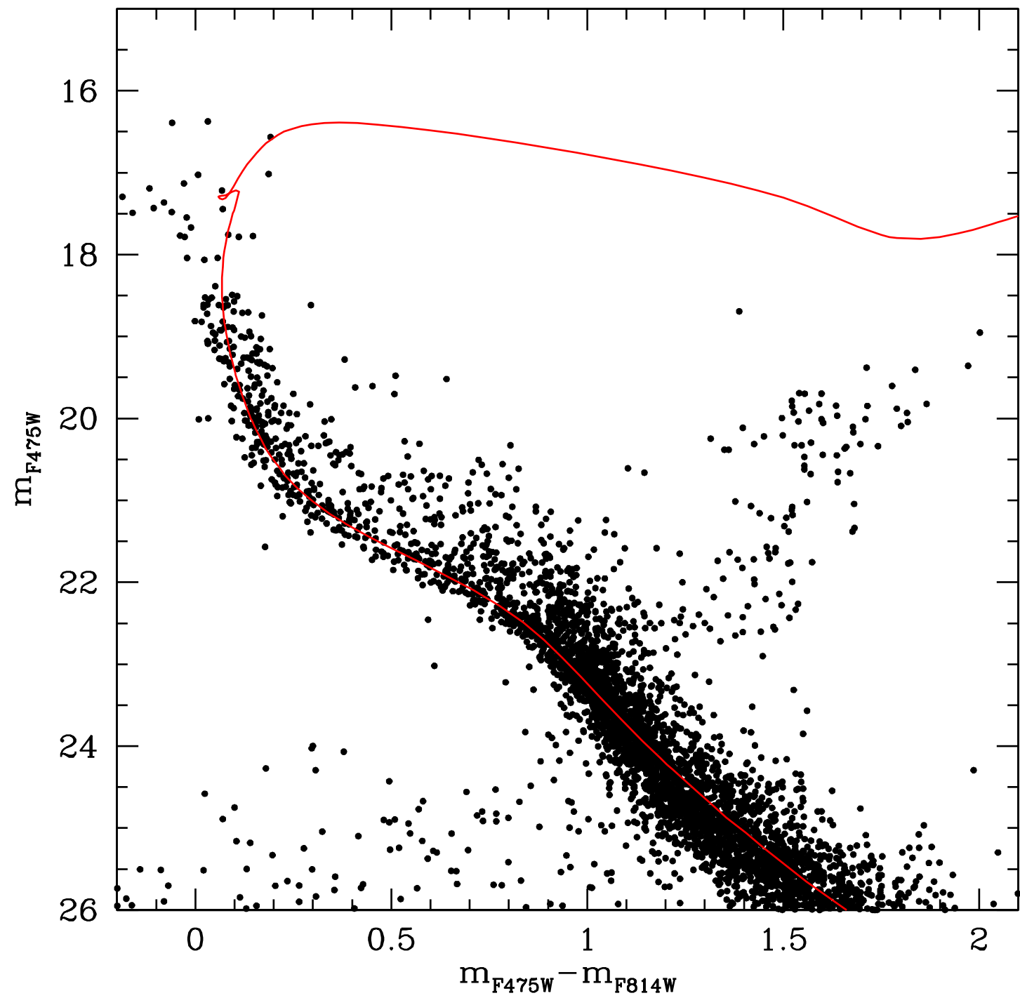
NGC 1793
