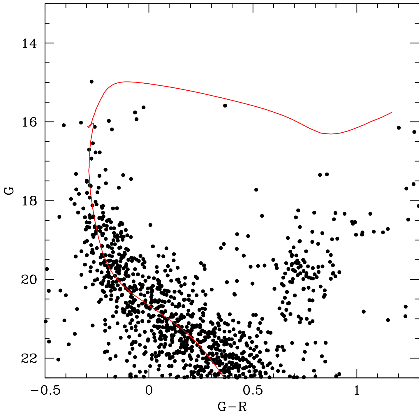
NGC 1834
