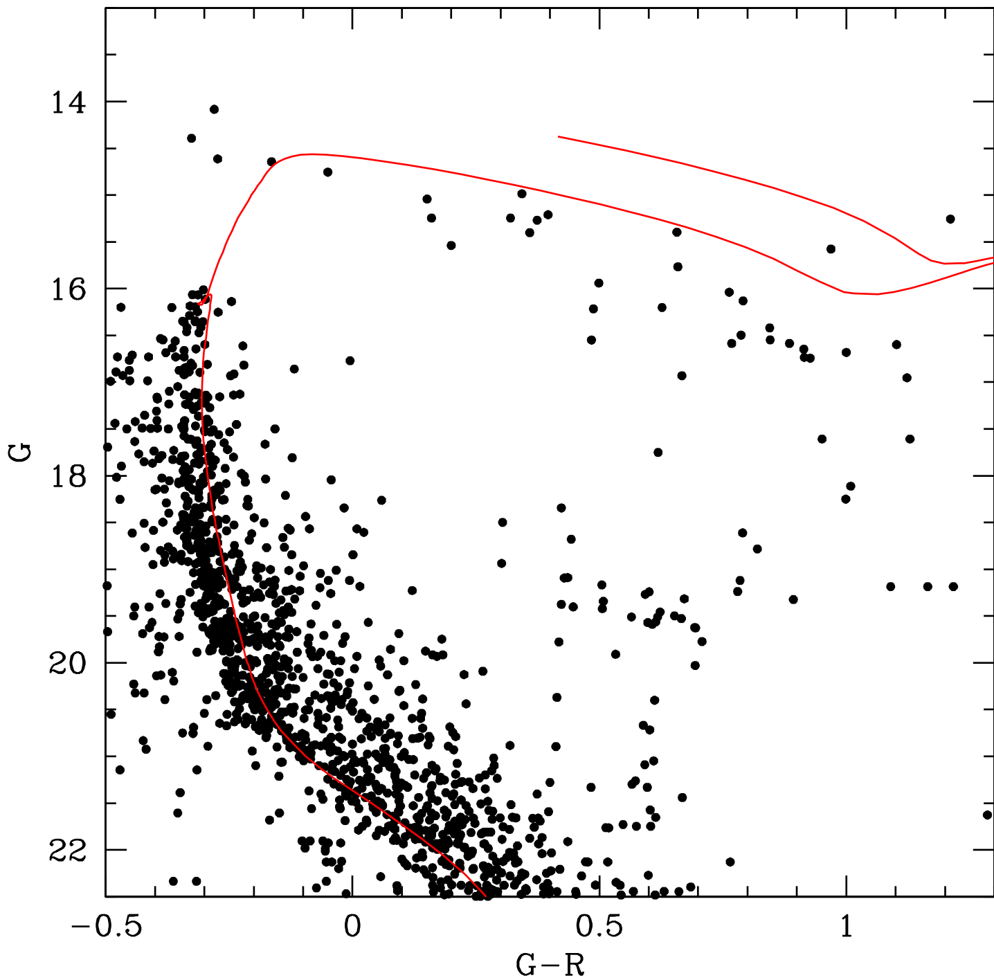
NGC 2041
