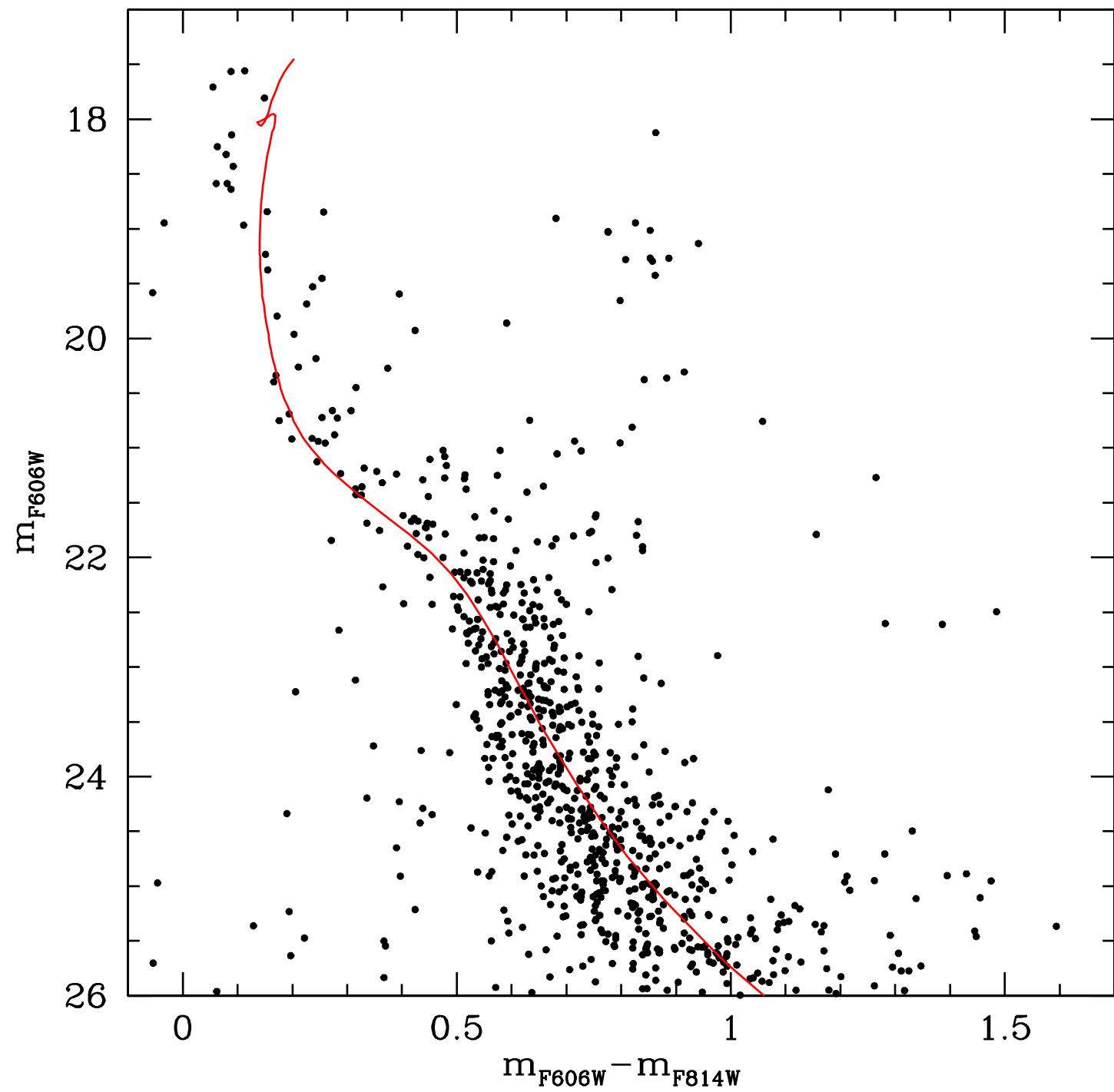
NGC 2091
