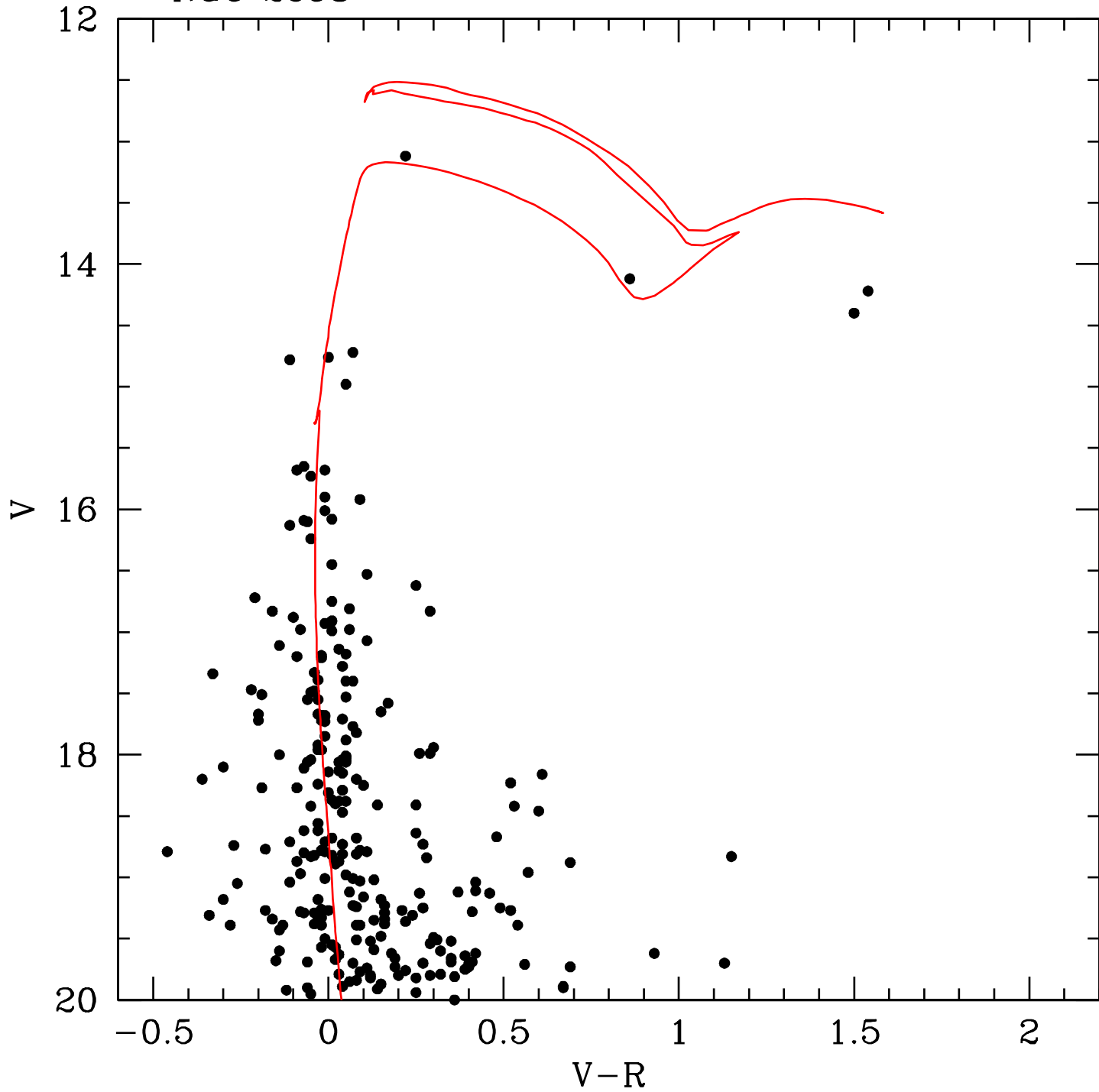
NGC 2098
