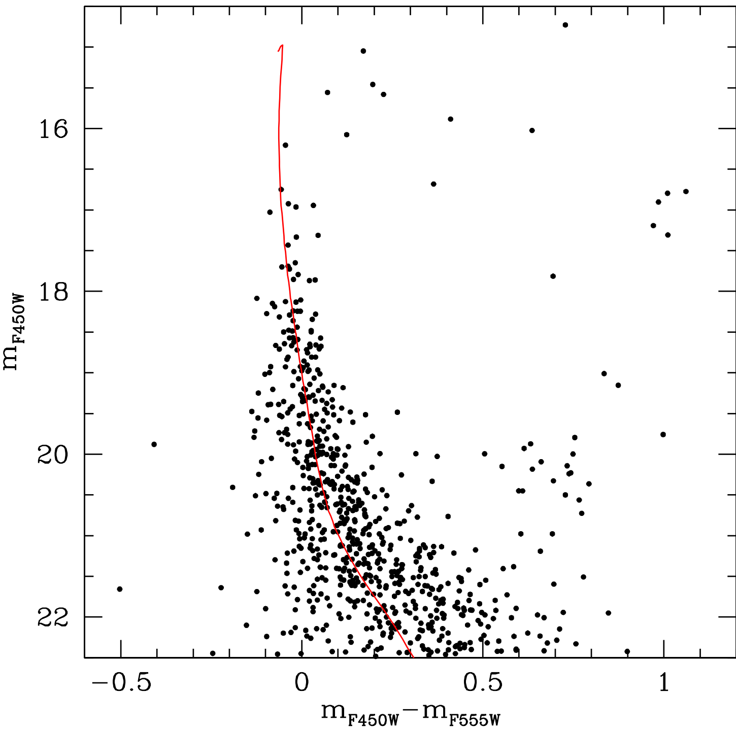
NGC 2136
