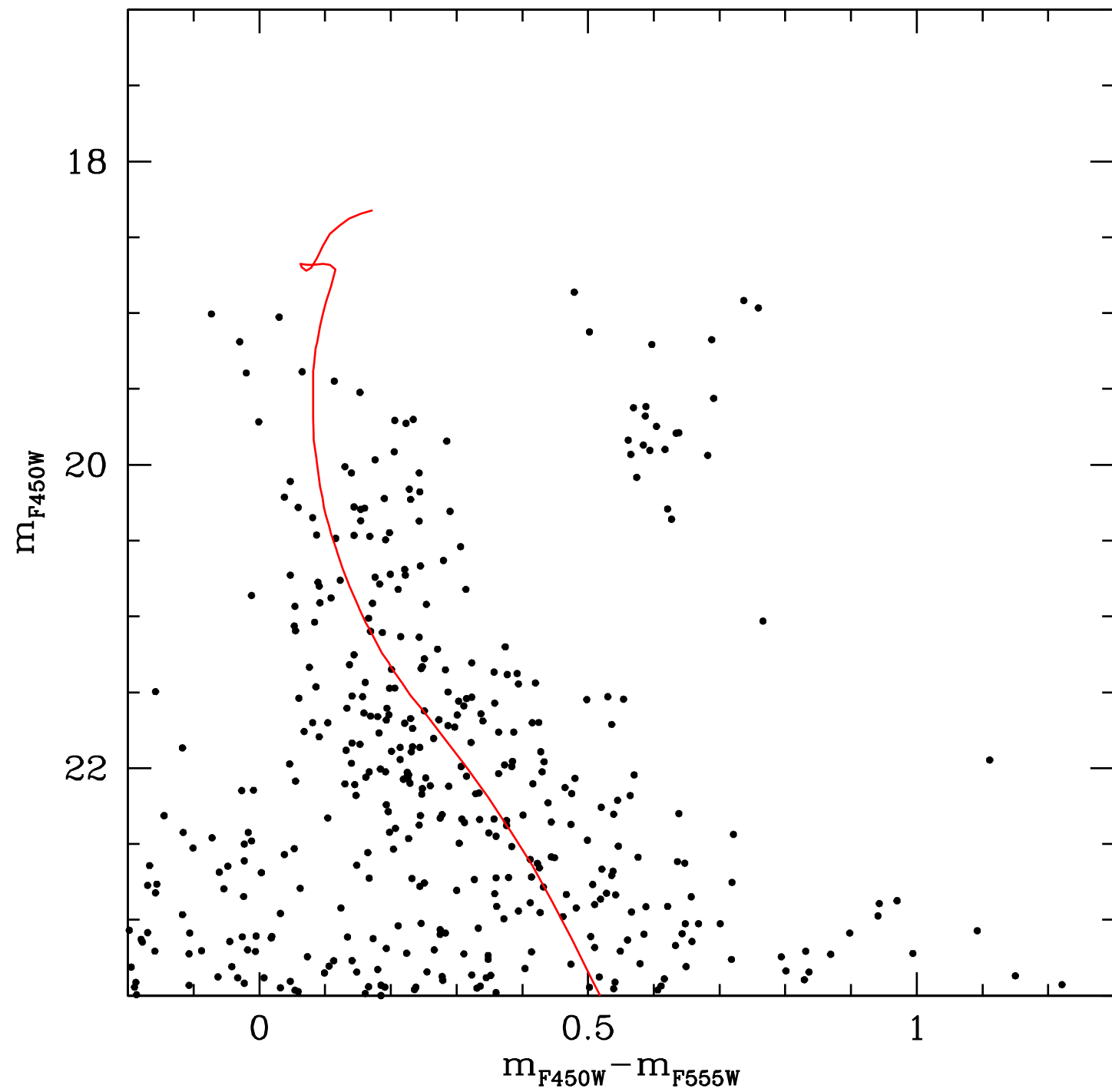
NGC 2153
