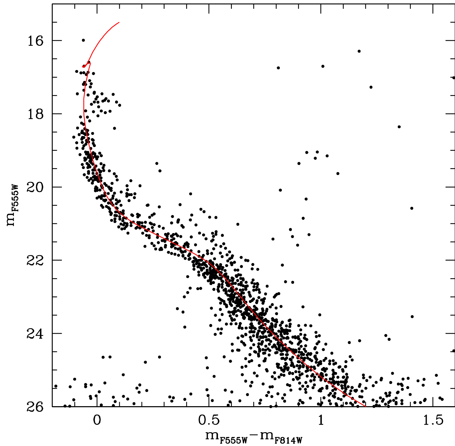
NGC 2159
