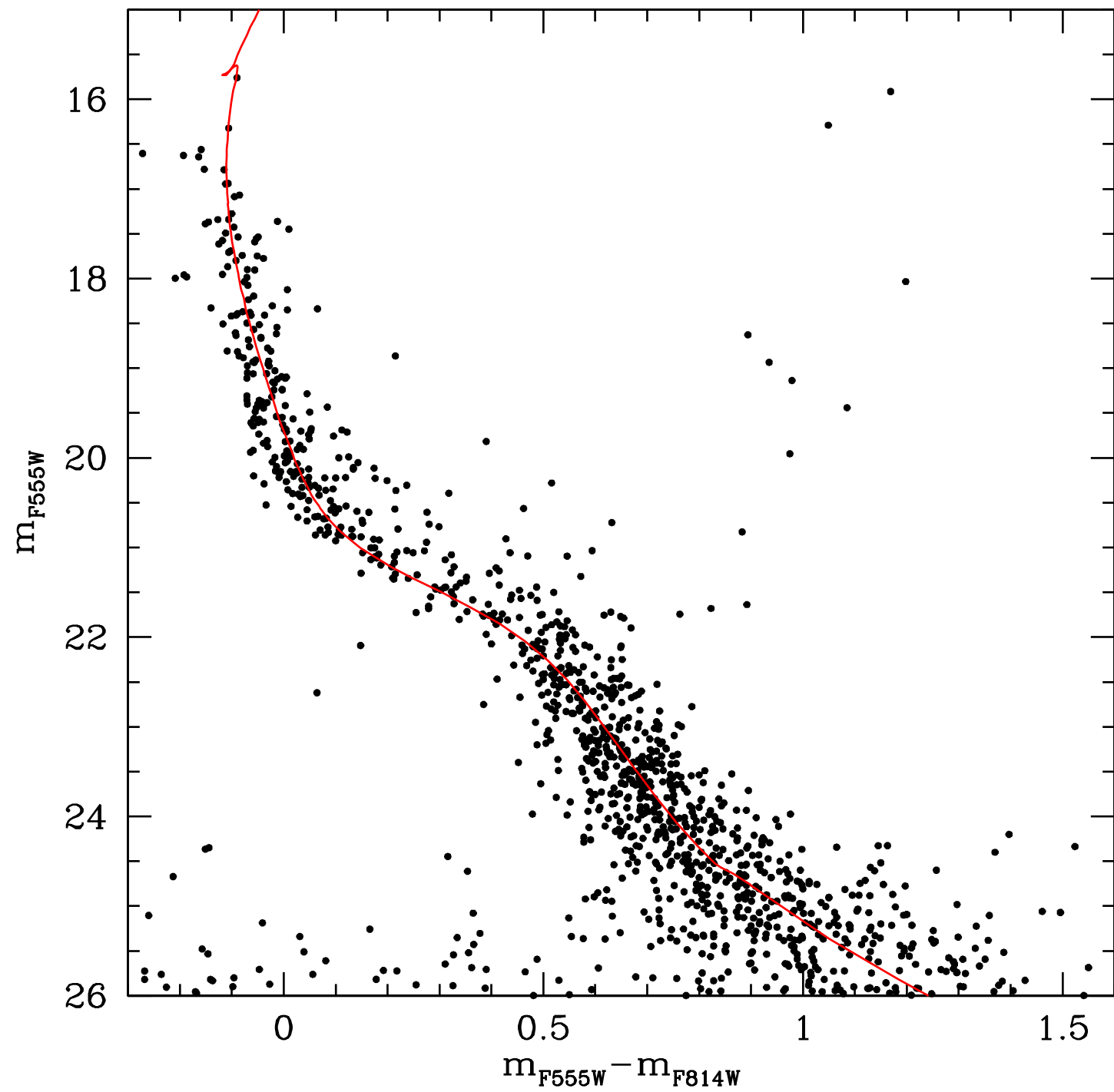
NGC 2172
