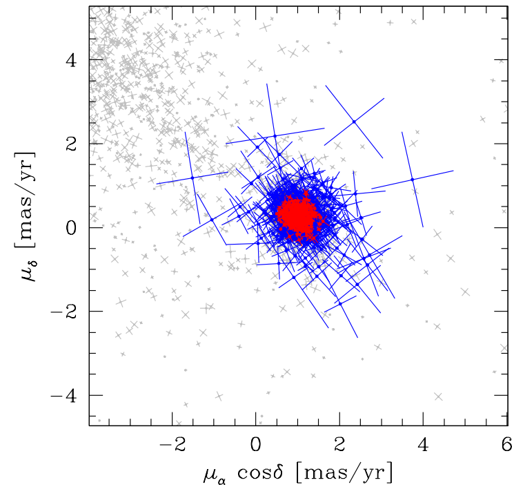
NGC 2808
