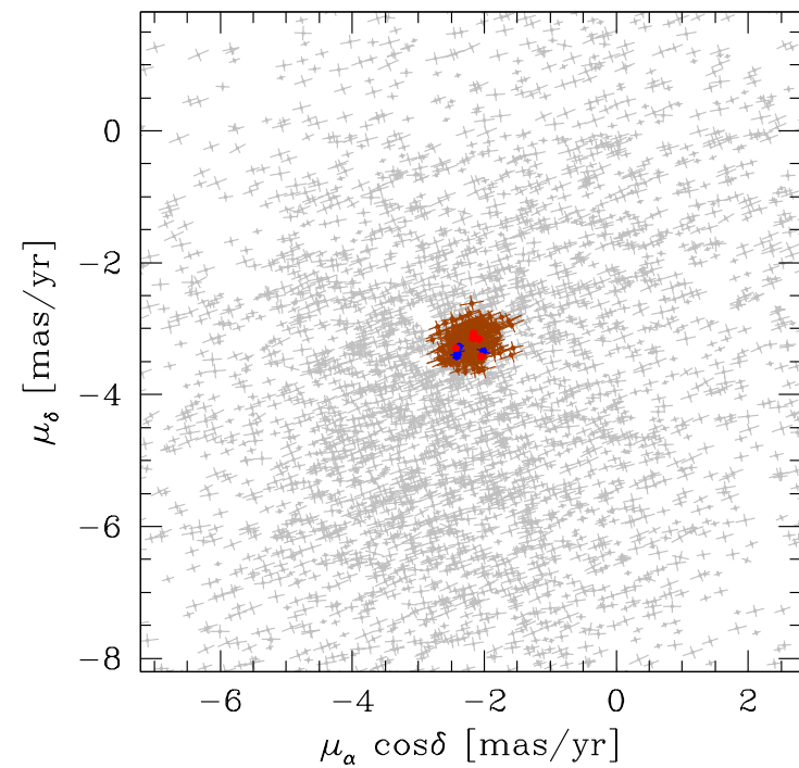
NGC 6333
